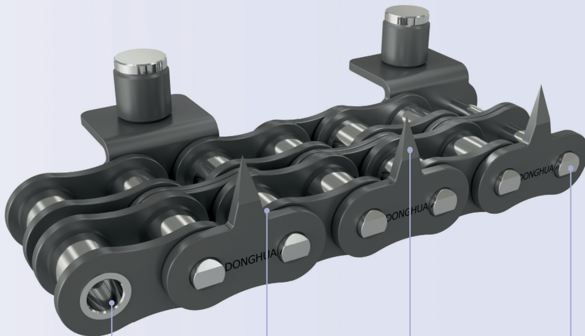
Keményített tüskék
