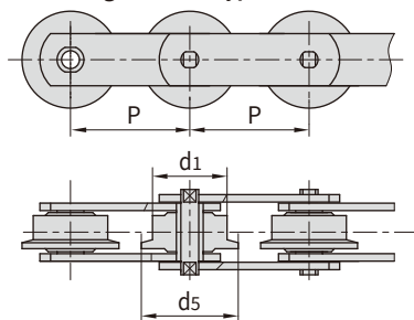
4.带F型带边滚子
